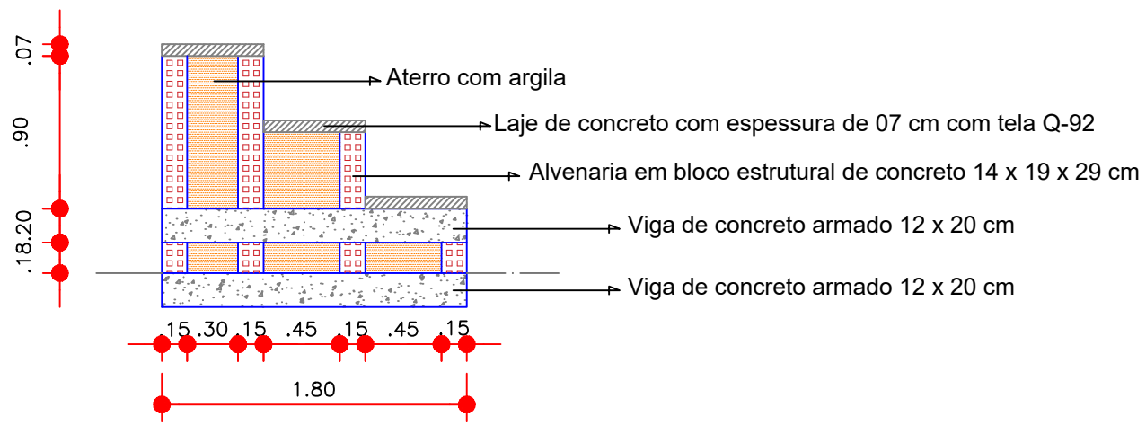
Corte AA'
