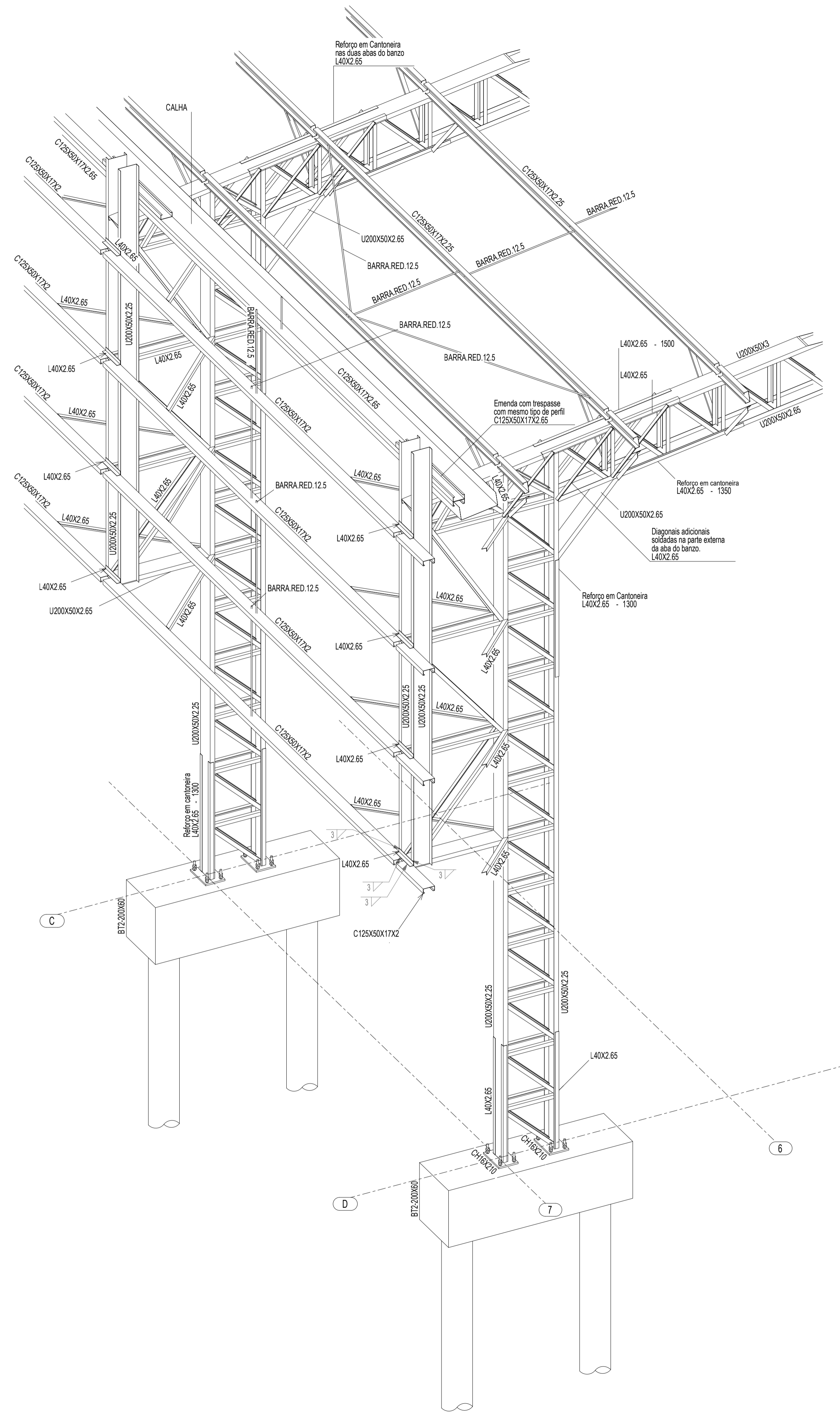
1 PERSPECTIVA DO EIXO 7C à 7D ESCALA 1/25
