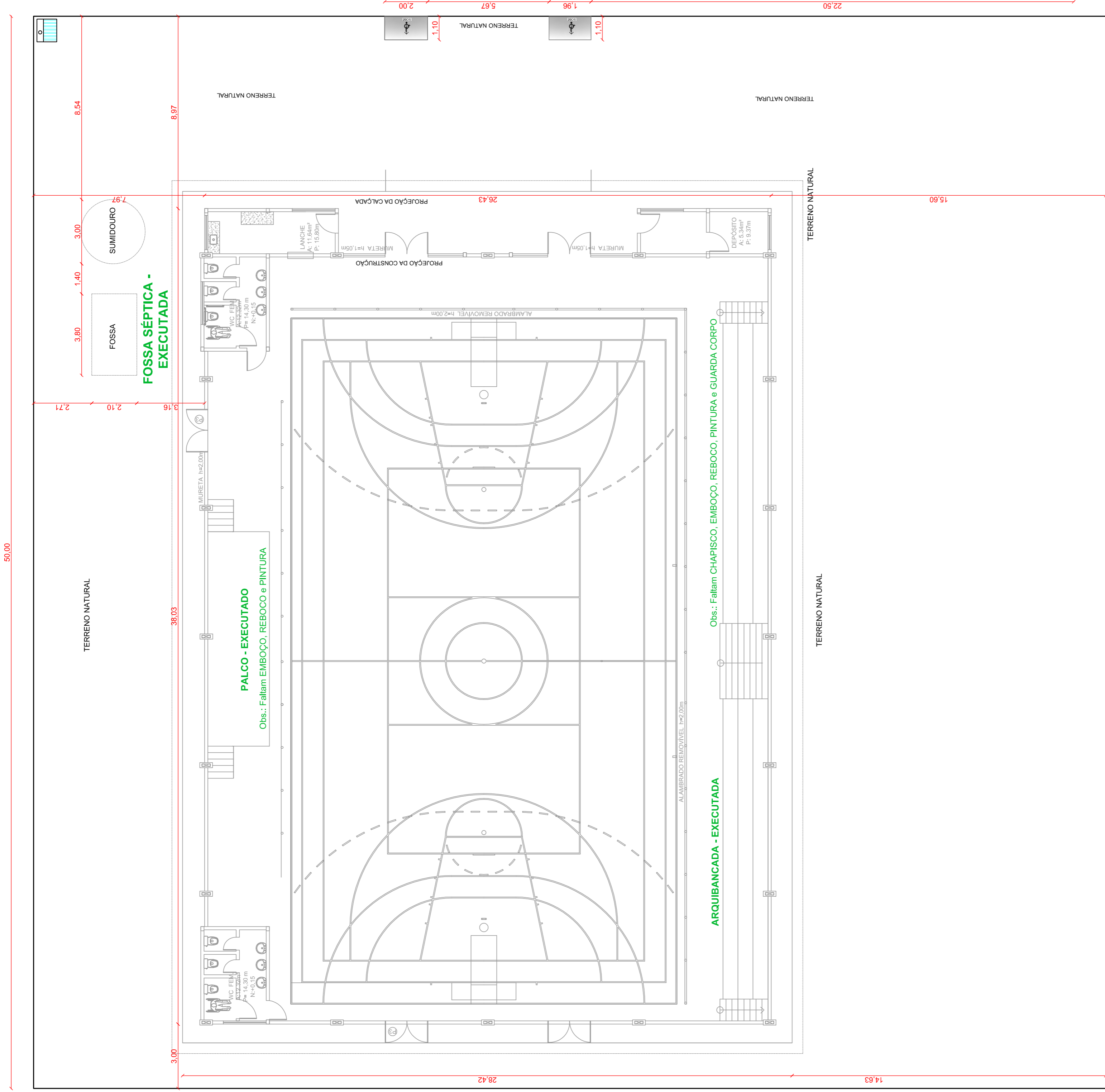
IMPLANTAÇÃO - COTAS ESCALA 1/125
