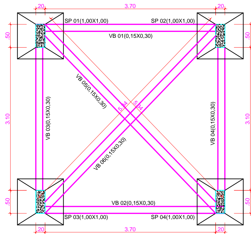
PLANTA DE INFRAESTRUTURA ESC. 1/50
