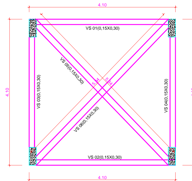
PLANTA DE SUPRAESTRUTURA ESC. 1/50
