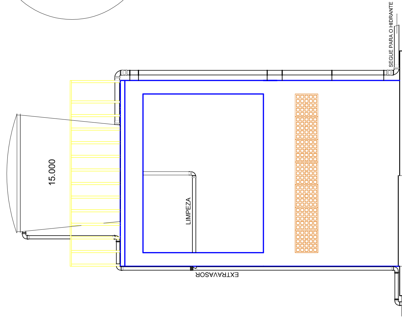
FACHADA 02 ESC. 1/50
