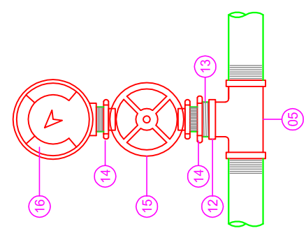
DET. 1 - MANÔMETRO S/ Esc.
