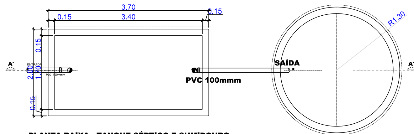
PLANTA BAIXA - TANQUE SÉPTICO E SUMIDOURO ESC. 1/50
