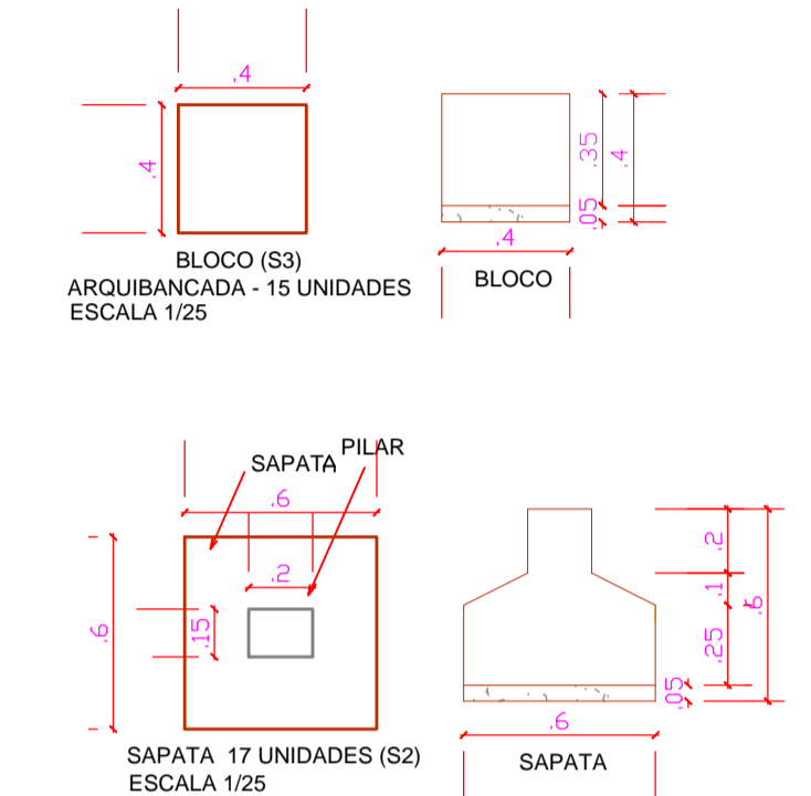
SAPATAS ESCALA 1/25
