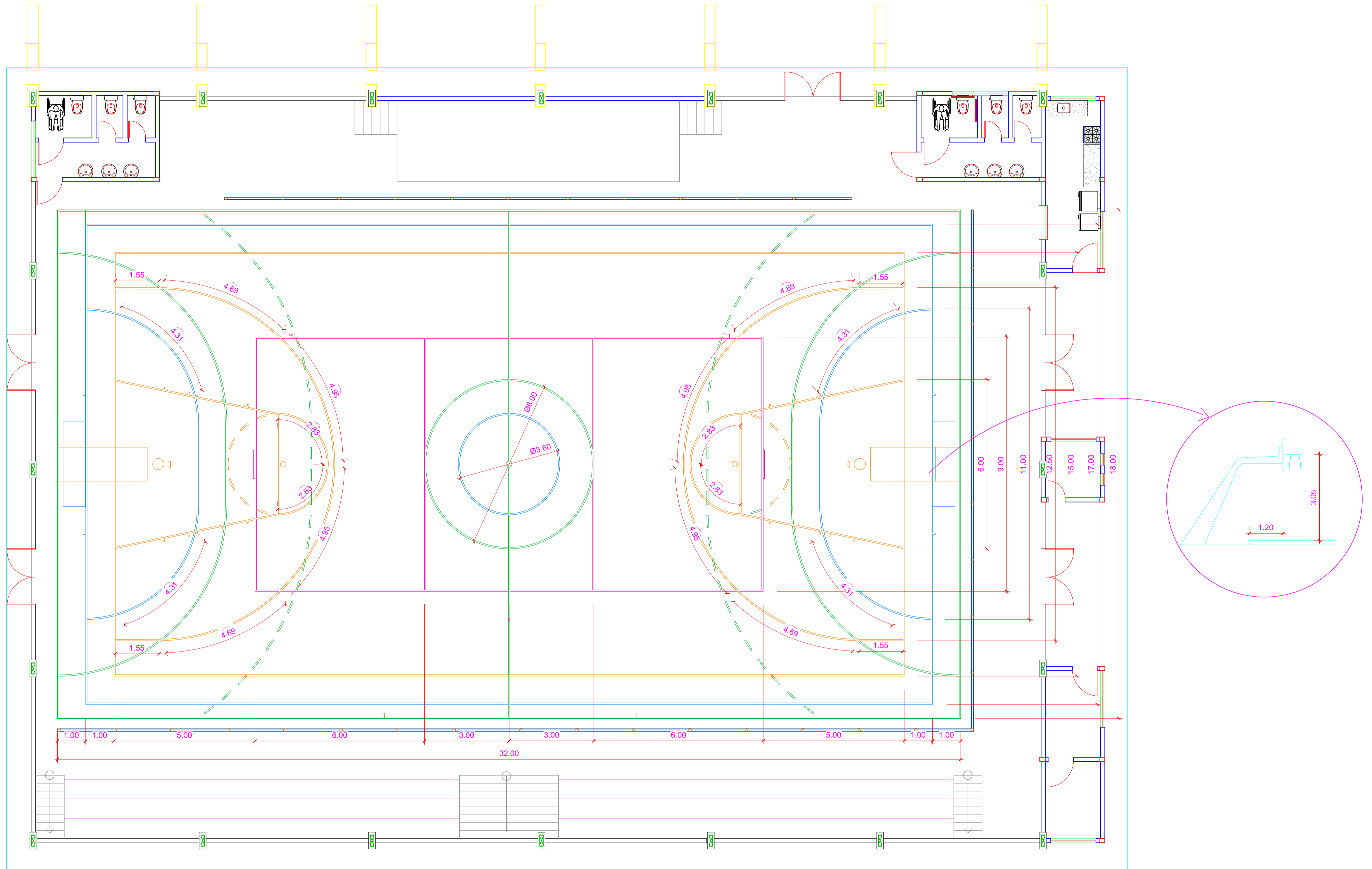
PLANTA DE DEMARCAÇÃO DE PISO ESCALA 1/75
