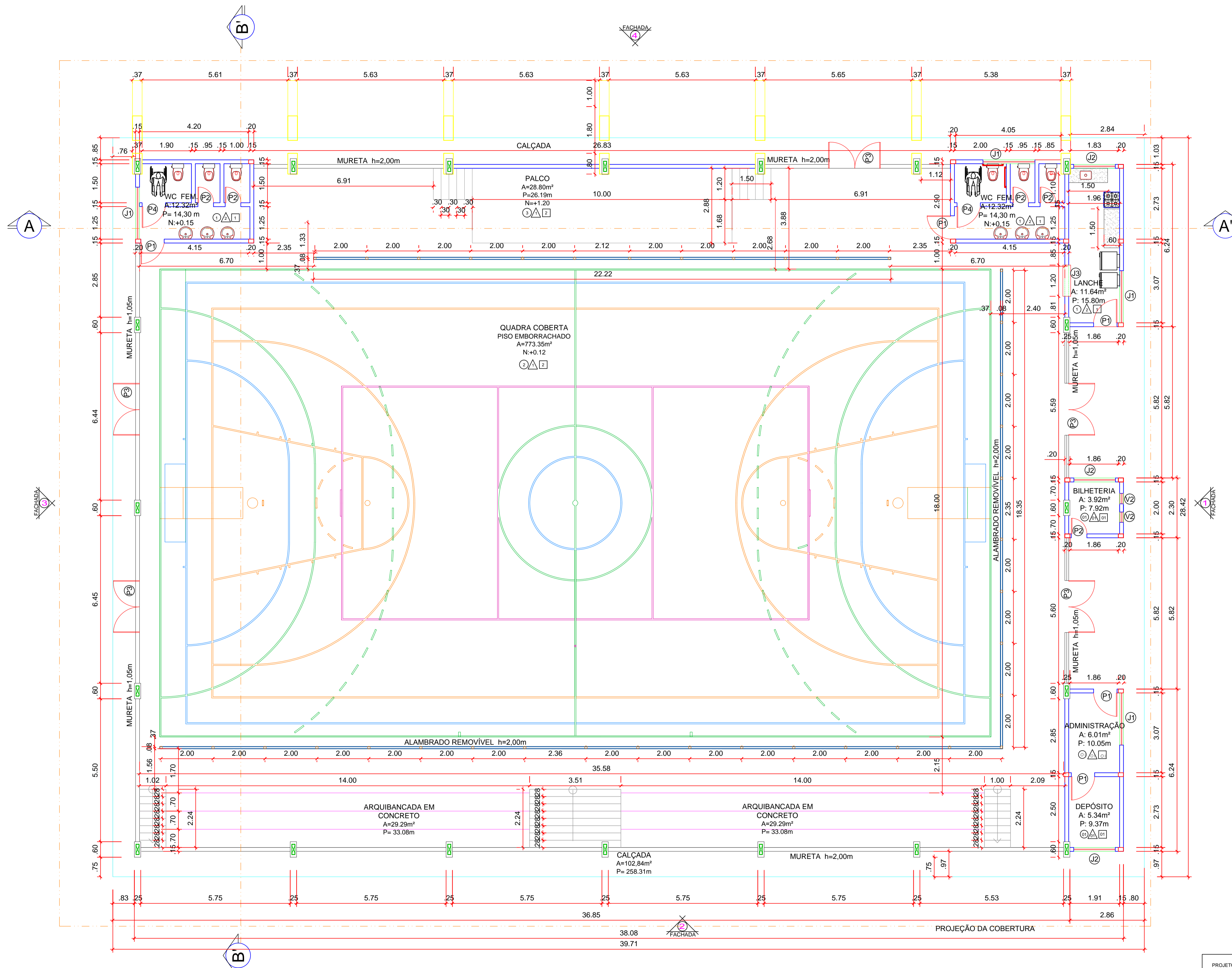
PLANTA BAIXA ÁREA CONSTRUÍDA: 991,06m² ESCALA: 1/75
