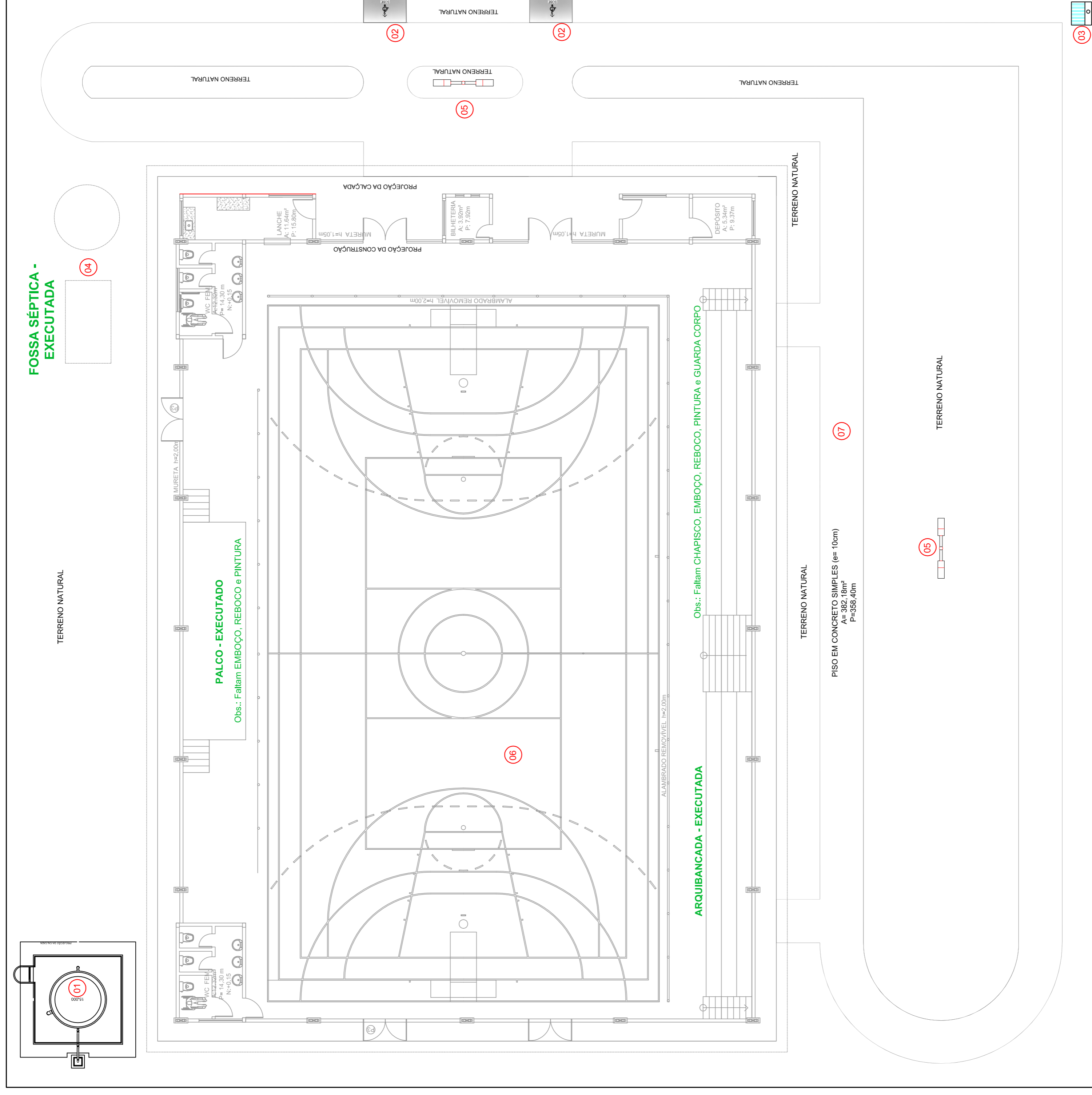
IMPLANTAÇÃO - LAYOUT ESCALA 1/125
