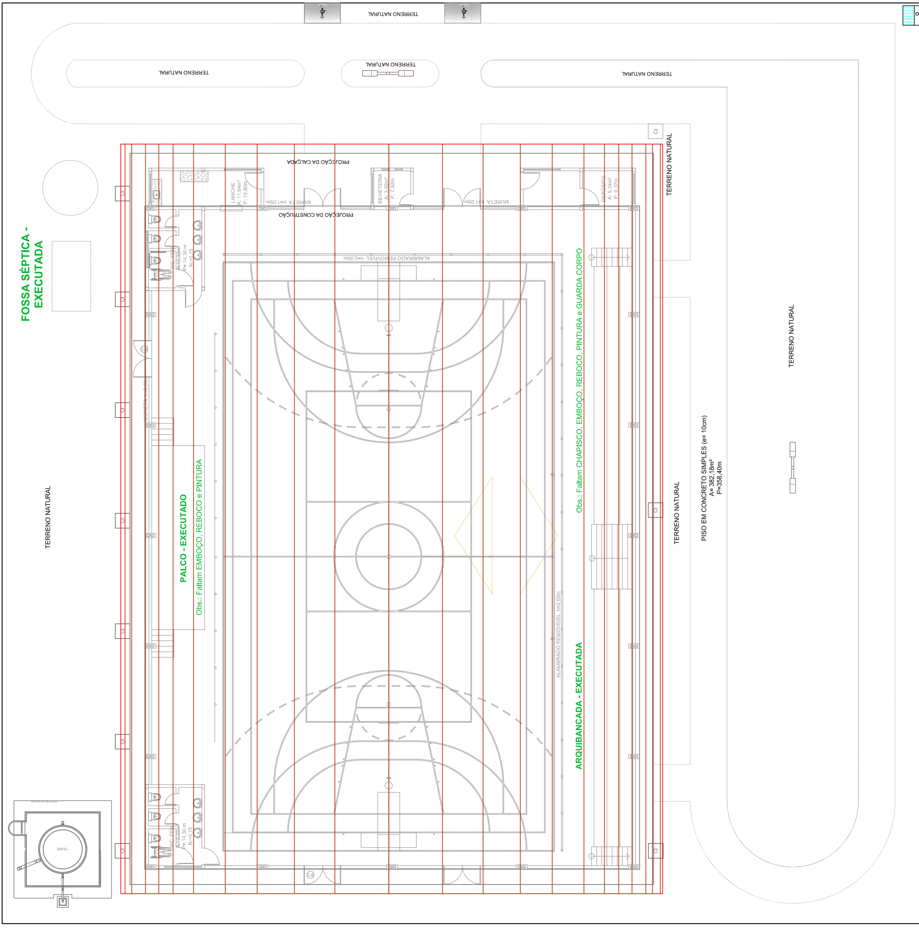
IMPLANTAÇÃO - COBERTURA DA QUADRA ESCALA: 1/125
