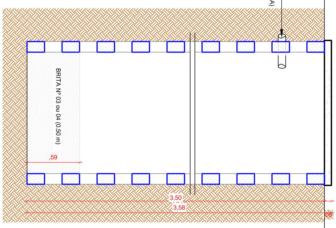
CORTE AA- SUMIDOURO ESC.: 1/25
